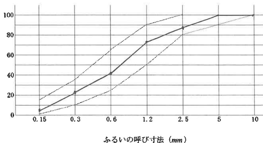
粒度曲線図
