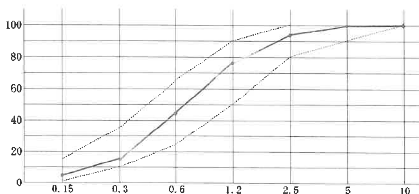
粒度曲線図
