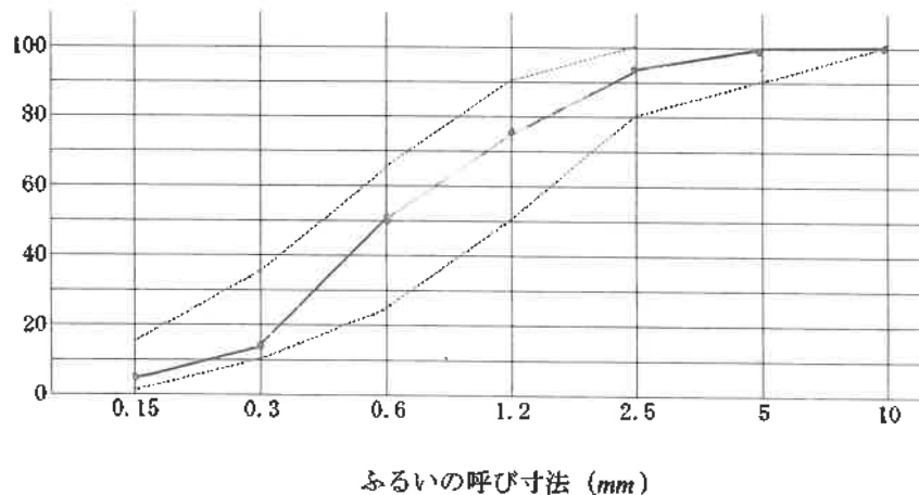
粒度曲線図
