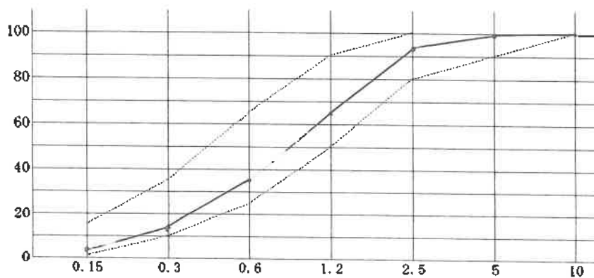
粒 度 曲 線 図
