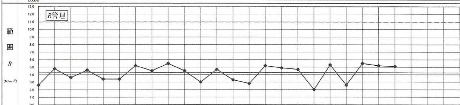
\bar{x} 管理図
