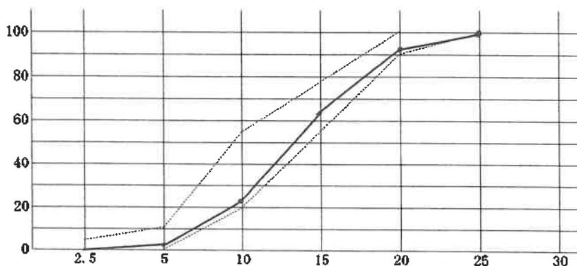
粒 度 曲 線 図
