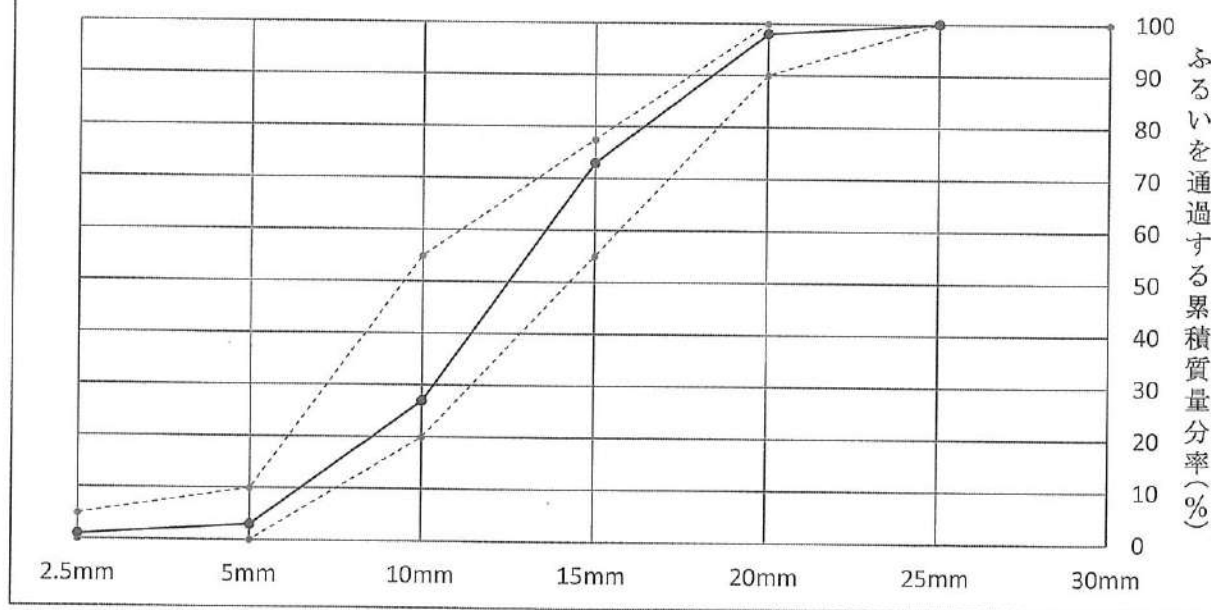
粒 度 曲 線
