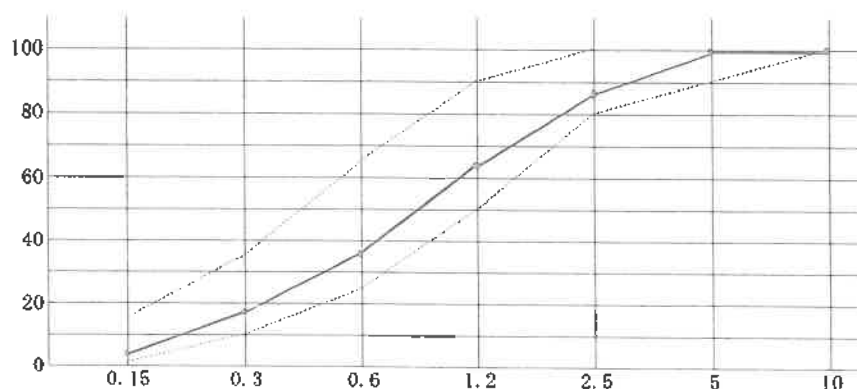
粒度曲線図
