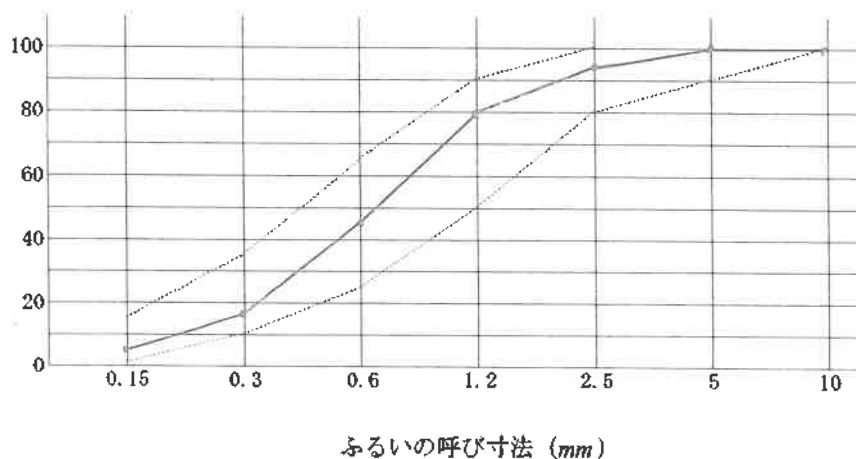
粒度曲線図
