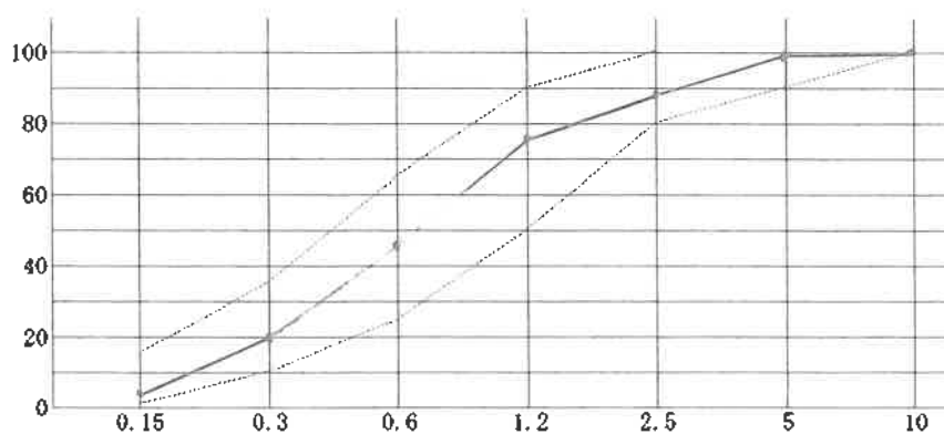
粒度曲線図
