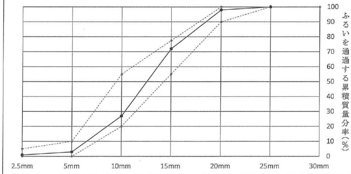
粒 度 曲 線
