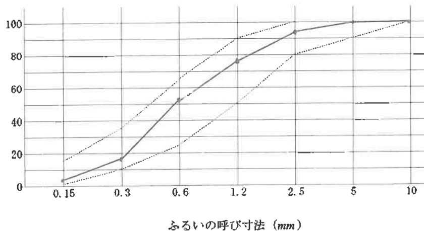
粒度曲線図
