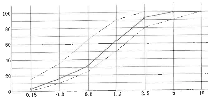
粒 度 曲 線 図
