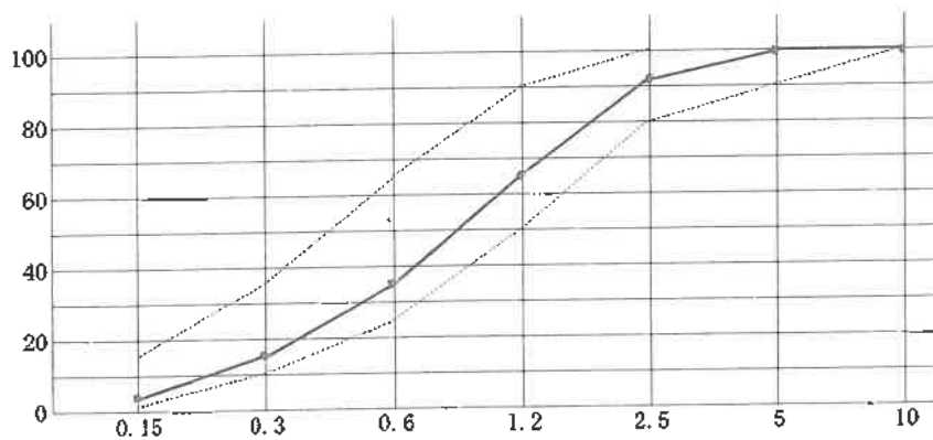
粒 度 曲 線 図
