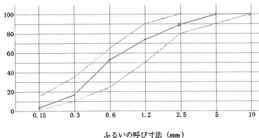
粒度曲線図
