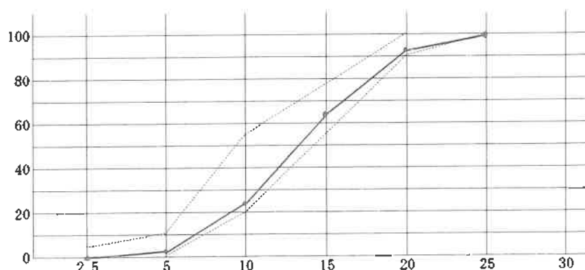
粒 度 曲 線 図
