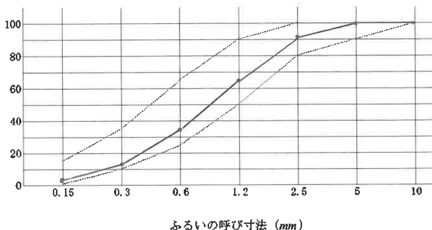
粒度曲線図
