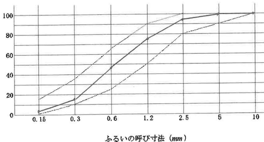
粒度曲線図
