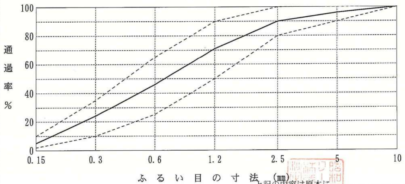
粒 度 曲 線
